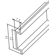
TH35-7.5 DIN rail
