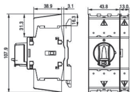
NF2-80/TS
