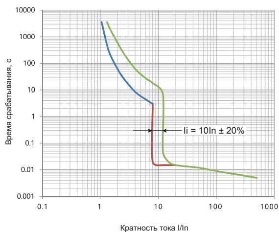
Времятоковая характеристика
