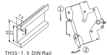
TH35-7.5 DIN Rail
