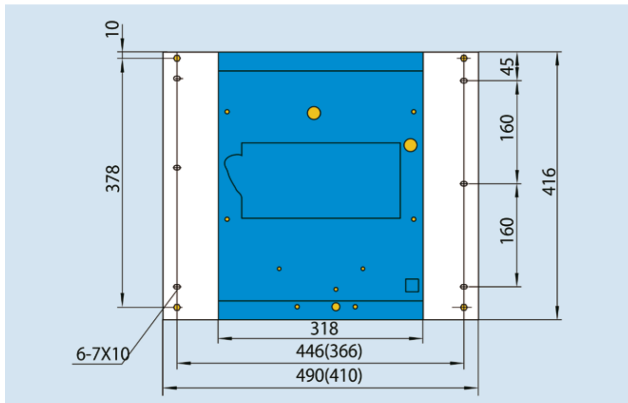
Рис. 6.3 Размеры выключателя с кабельной муфтой
